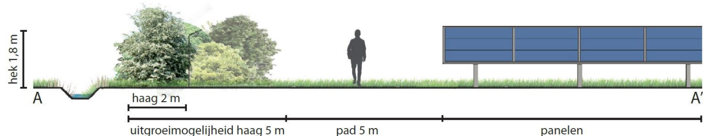
Principedoorsnede haag westzijde plangebied A - A'
